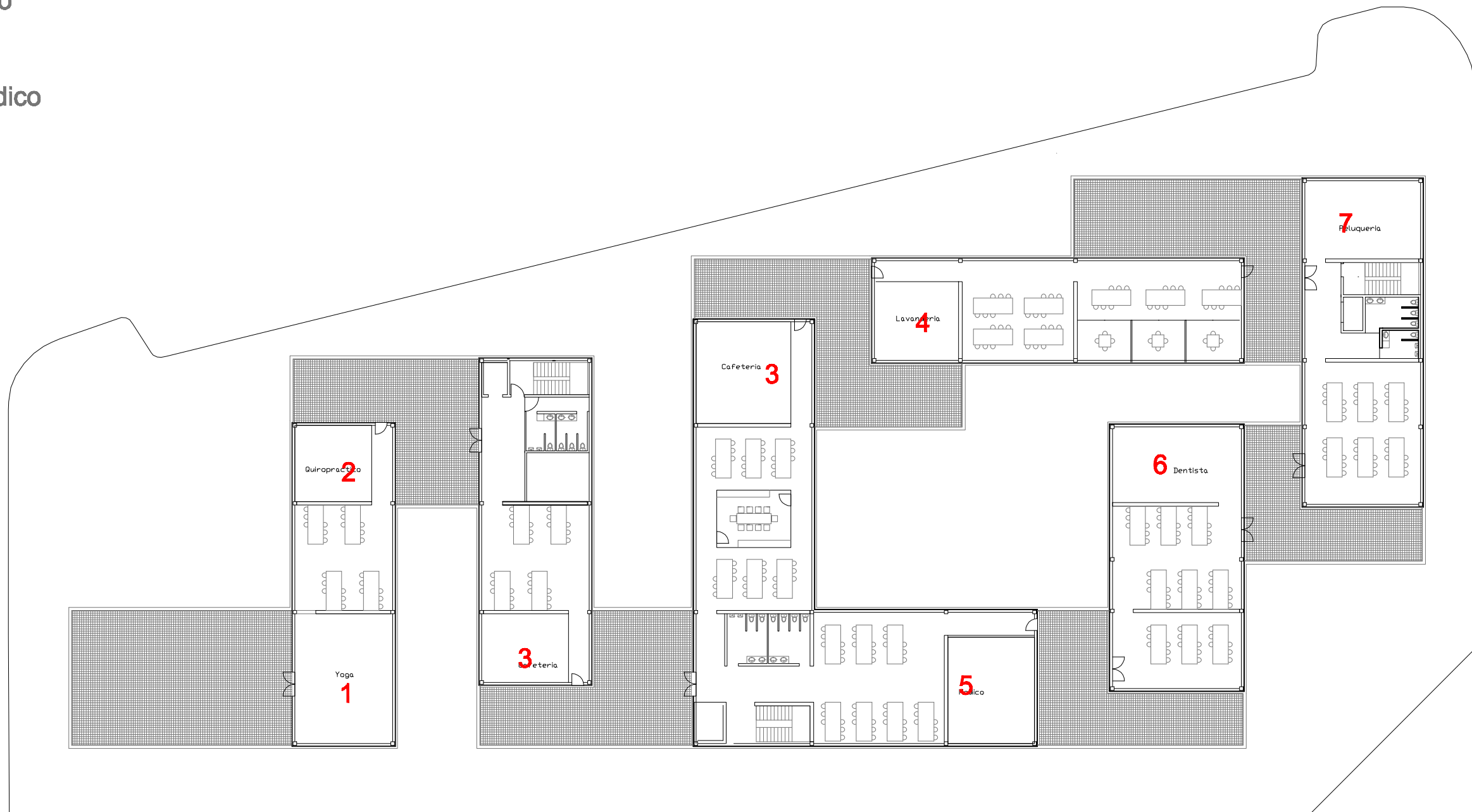
Planta 1ª(oficina_servicios) 1:200
