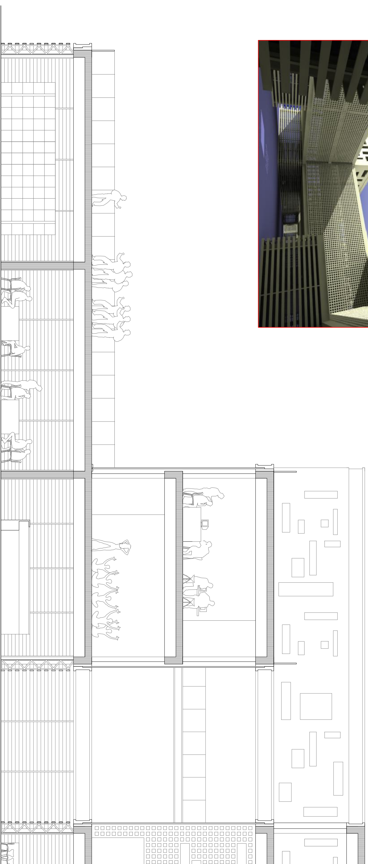
SECCION CONSTRUCTIVA 1:100
